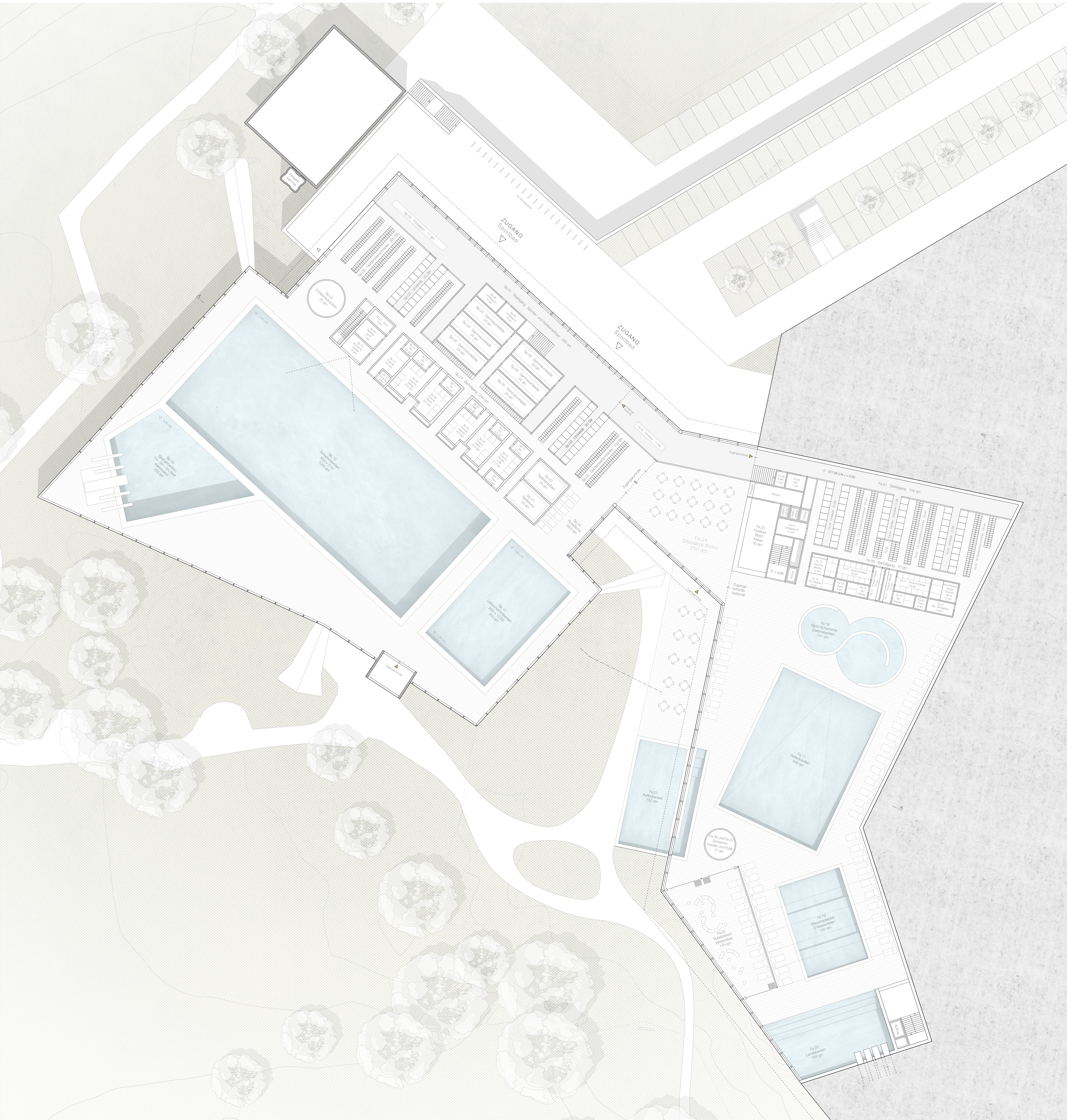
Grundriss Sockelgeschoss 1:200
